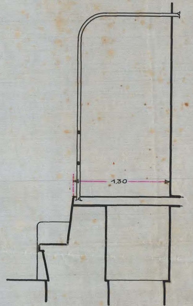
SECCION
