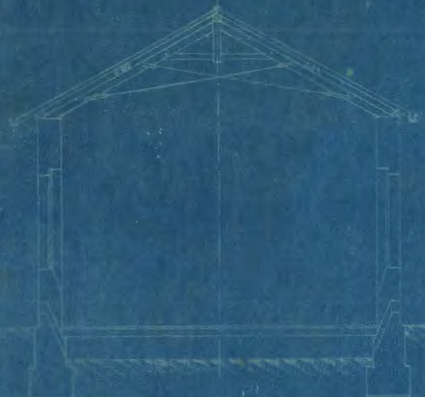
Seccion E.F.
